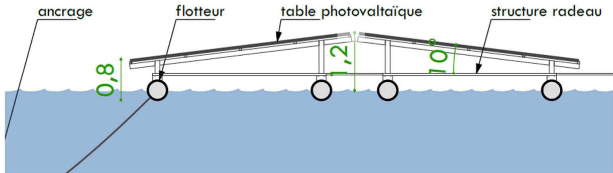
Panneau Photovoltaïque Flottant
